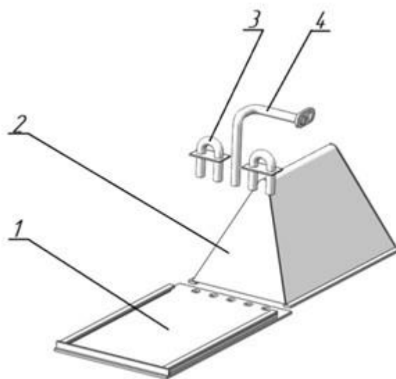
Рисунок 31 – Общий вид колёсного упора
