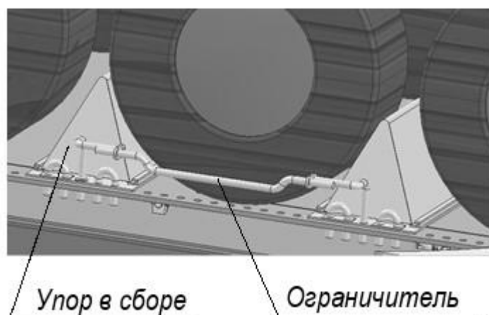
Рисунок 34 – Крепление колеса колёсными упорами
