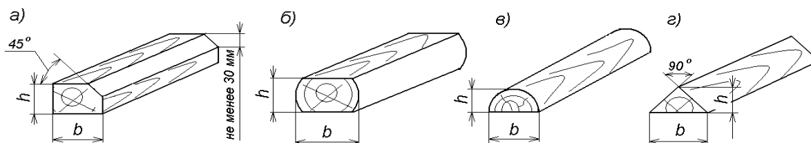
Рисунок 7 – Варианты исполнения упорных брусков для подклинивания обремененных колес из:
