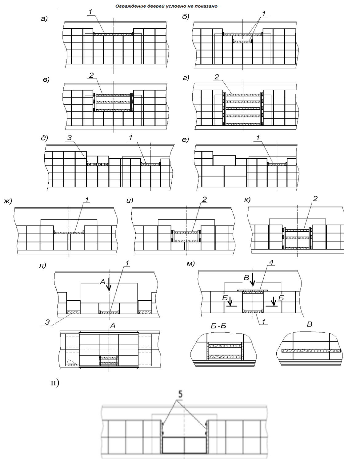
Рисунок 15 – Примеры крепления ящиков, пакетов в продольном направлении 1 – распорная рама; 2 – распорная конструкция; 3 – подкладка; 4 – накладка-распорка; 5 – щит
