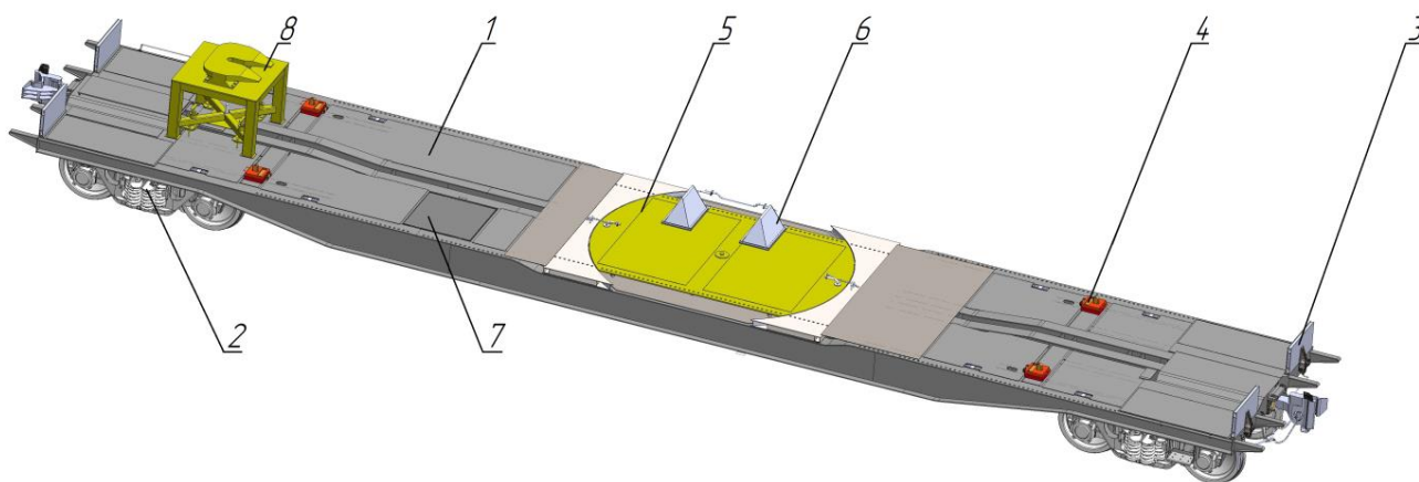
Рисунок 5а – Платформа модели 13-9938
