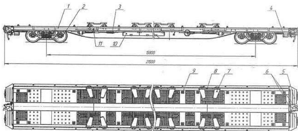
Рисунок 1 – Платформа модели 13-9961
