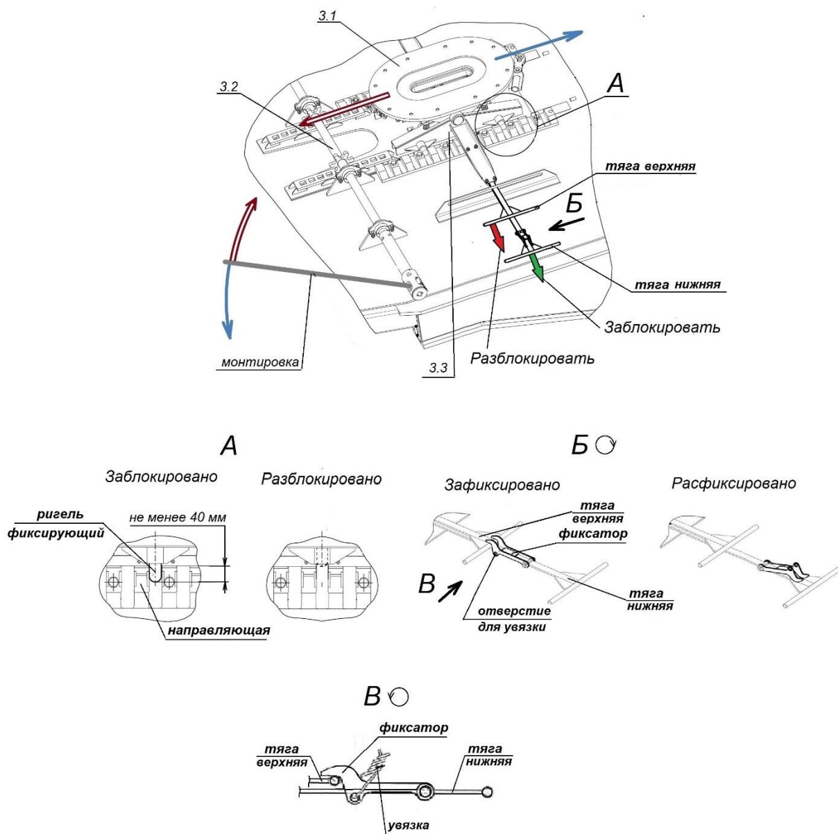
Рисунок 37 – Устройство опорное
