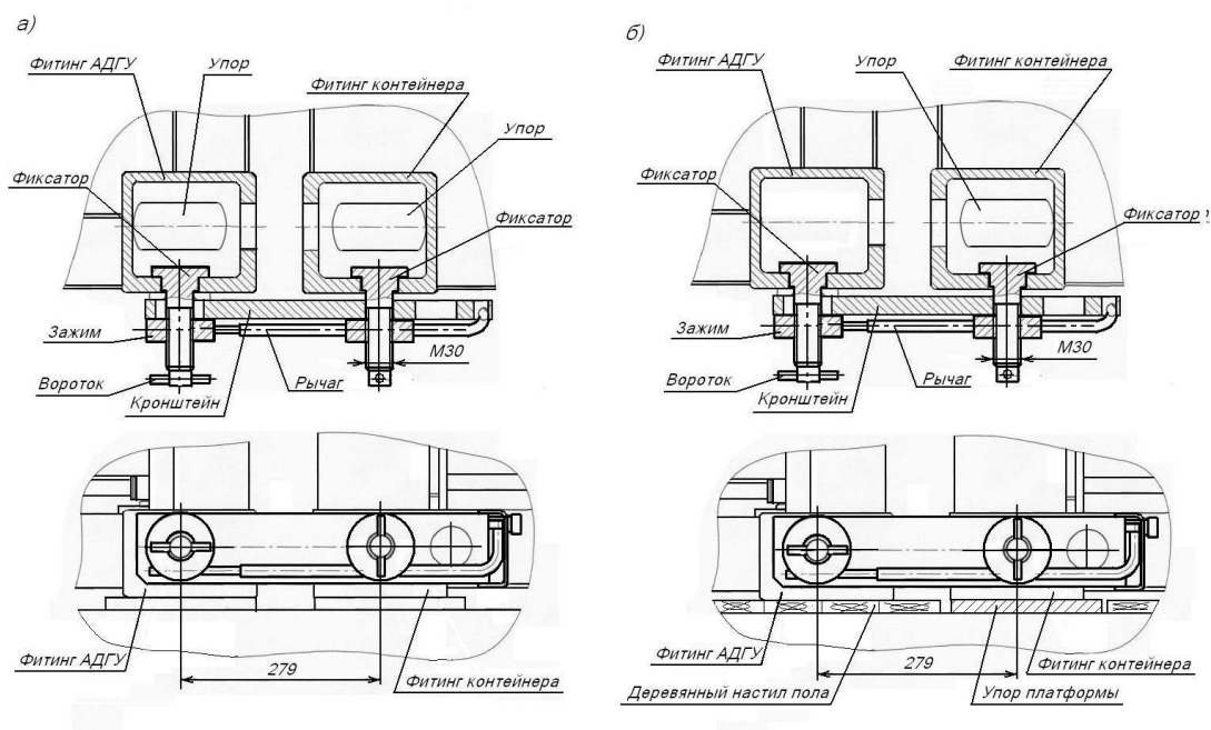
Рисунок 20 а – на платформе без деревянного настила пола; б – на платформе с деревянным настилом пола
