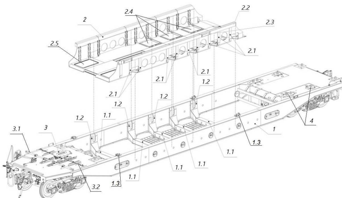
Рисунок 36 – Схема взаимного положения рамы и поддона
