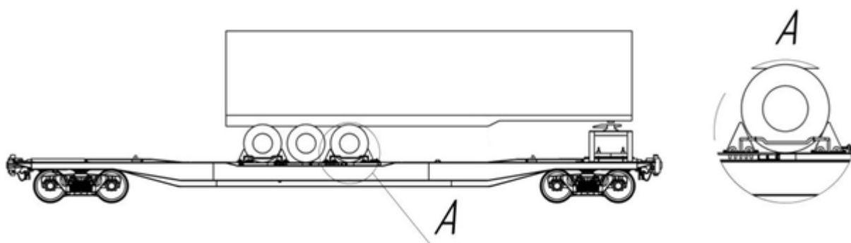
Рисунок 33 – Размещение и крепление полуприцепа на платформе модели 13-9938
