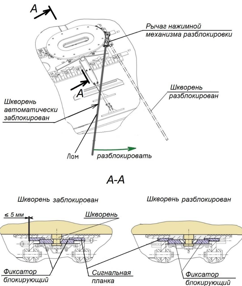
Рисунок 38 Блокировка и разблокировка шкворня полуприцепа
