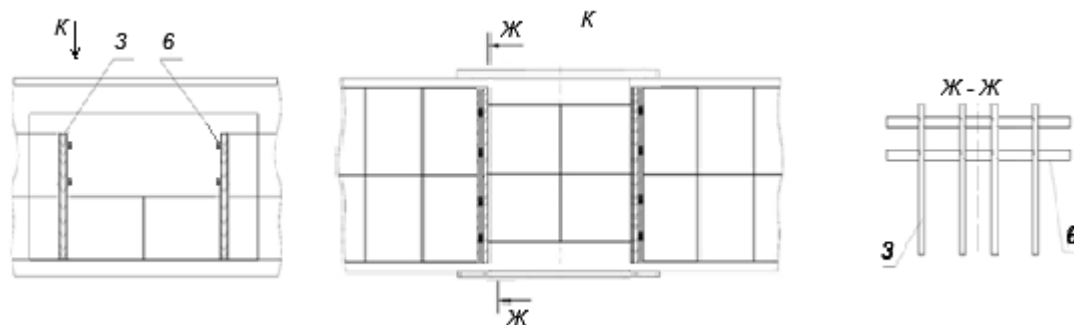
Рисунок 16 – Распорная рама, распорная конструкция, щит 1 – упорная доска; 2 – распорный брусок; 3 – стойка; 4 – брусок; 5 – накладка; 6 – доска; 7, 8 – опорные бруски
