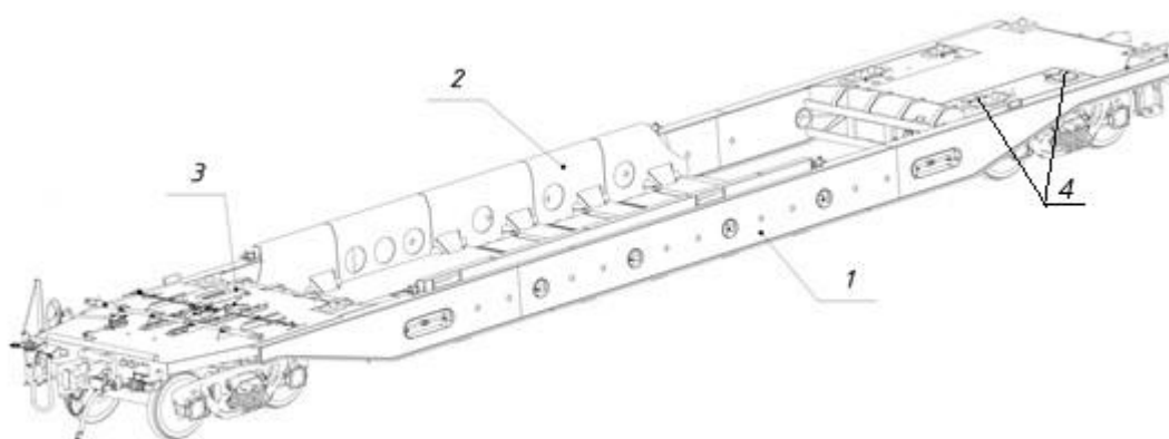
Рисунок 5б – Платформа модели 13-6701
