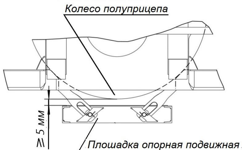
Рисунок 41 – Схема контроля положения колес полуприцепа, относительно площадки опорной подвижной.
