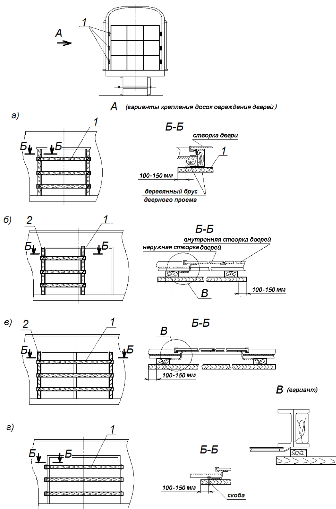
Рисунок 3 – Варианты ограждения дверей 1 – горизонтальная доска; 2 – стойка
