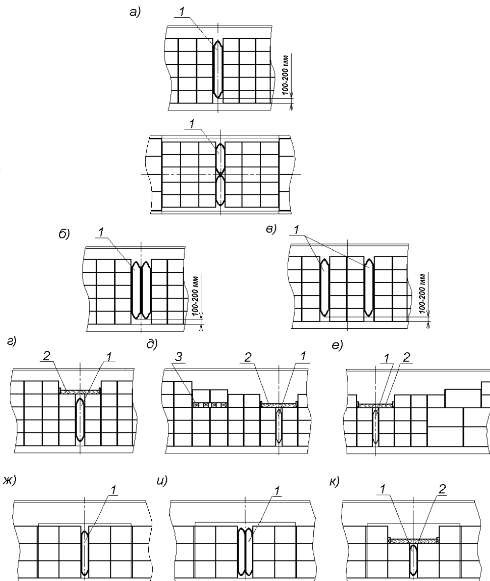
Рисунок 17 – Примеры крепления ящиков, пакетов в продольном направлении с использованием пневмооболочек
