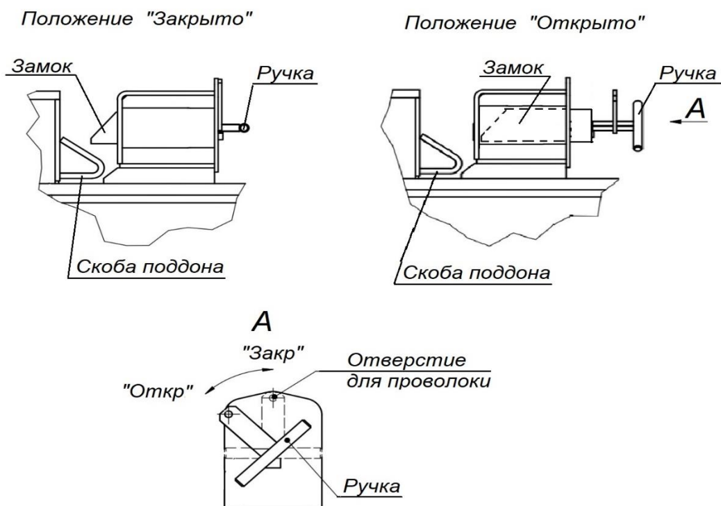
Рисунок 43 - Положения фиксаторов поддона
