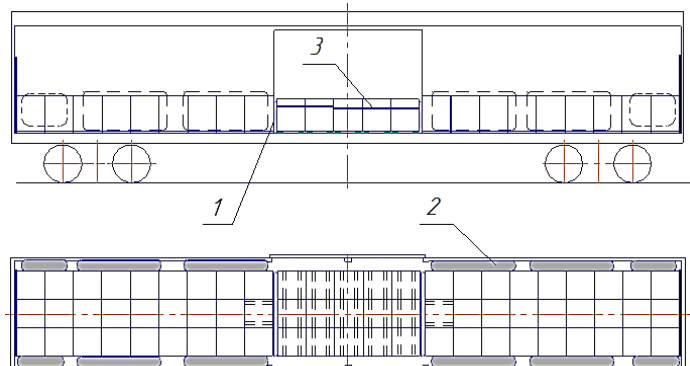
Рисунок 39 – Размещение слитков алюминия, сформированных в пакеты, в один ярус 1 - пневмооболочки 100 х 220 см или 85 х 220 см; 2 – пневмооболочки, закрепляющие от поперечных смещений; 3 – увязка
