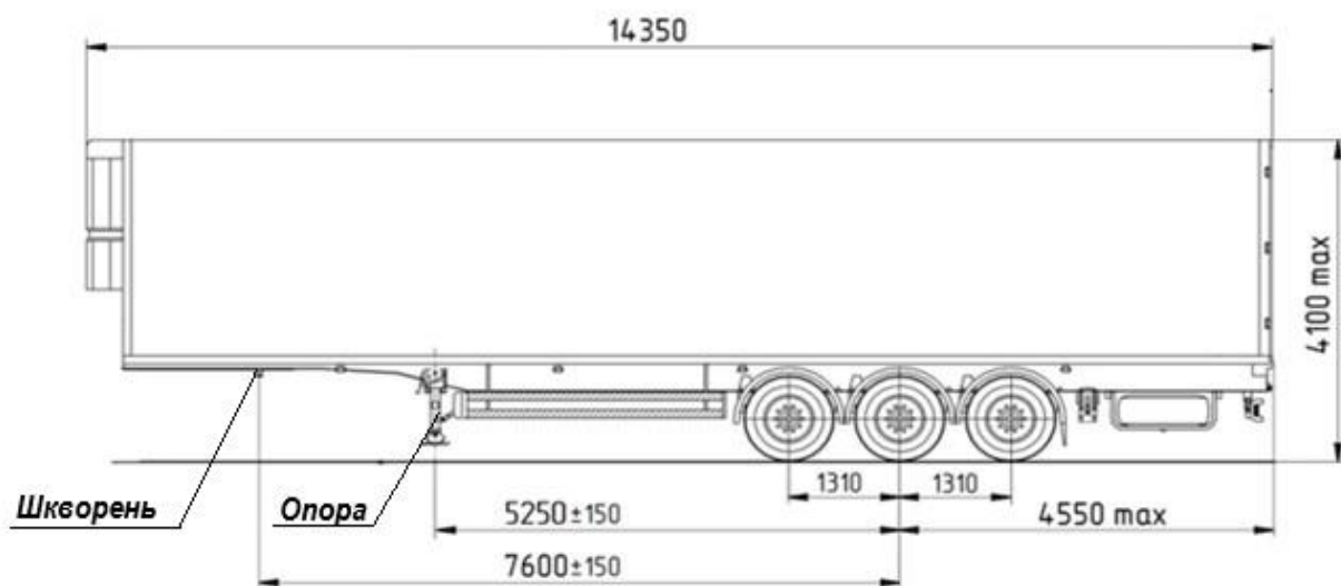
Рисунок 35 – Основные геометрические размеры полуприцепов
