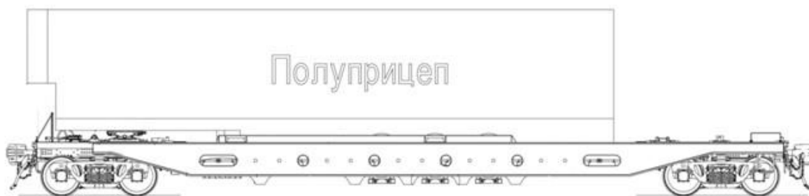
Рисунок 39 – Схема размещения полуприцепа на платформе модели 13-6701
