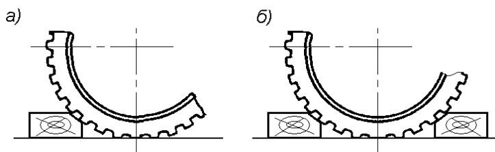
Рисунок 6 – Подклинивание обремененных колес техники а – с одной стороны; б – с двух сторон
