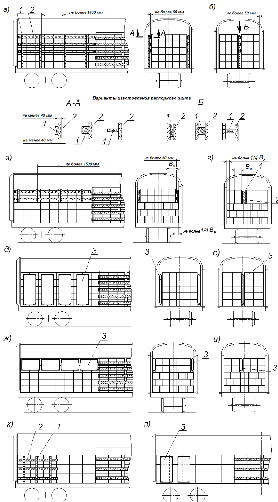
Рисунок 18 – Примеры крепления ящиков, пакетов в поперечном направлении:
