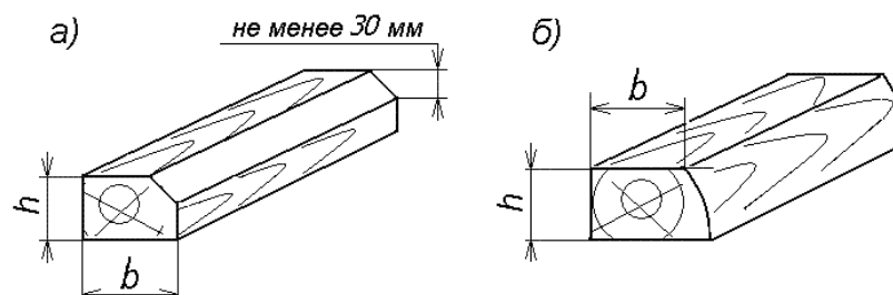
Рисунок 8 – Варианты исполнения поперечных упорных брусков:
