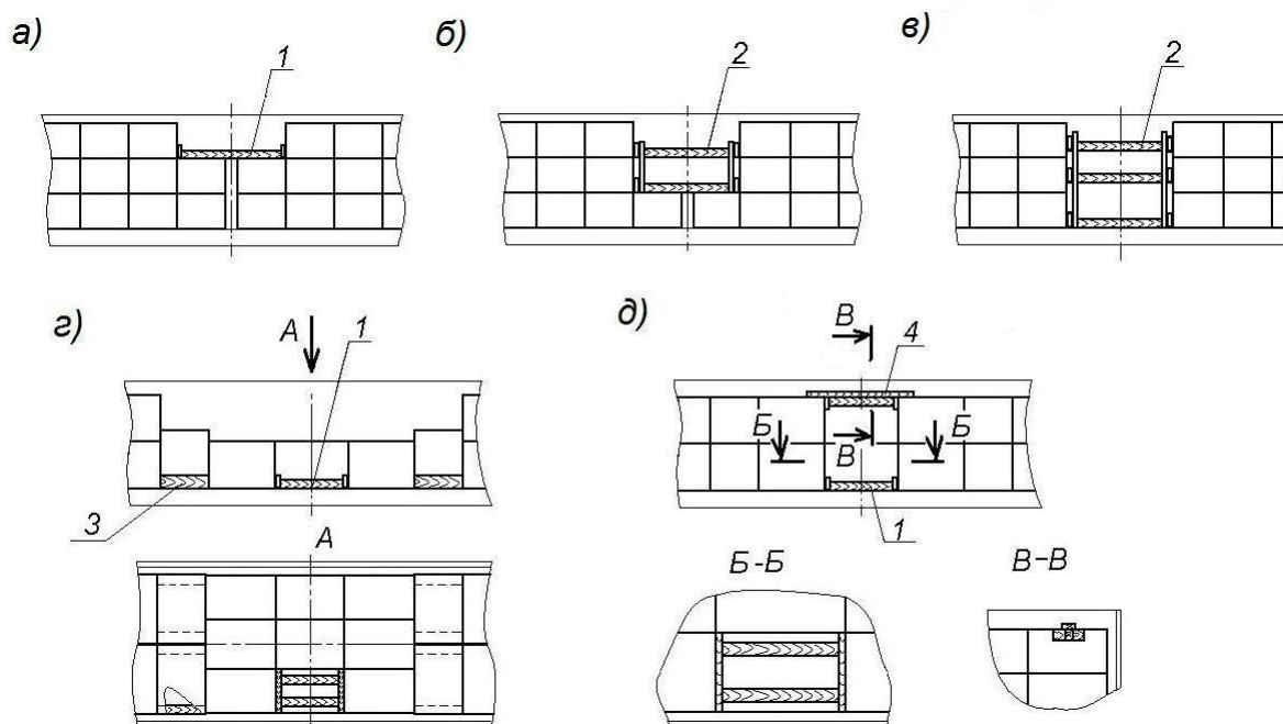
Рисунок 4 – Примеры крепления пакетов в продольном направлении
