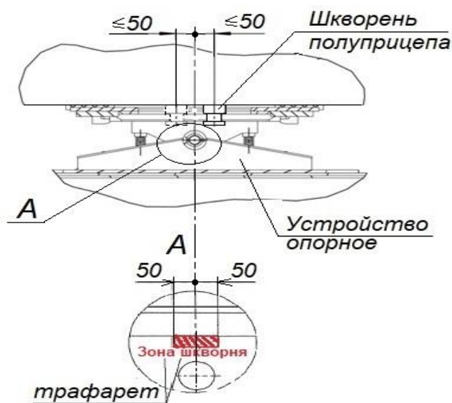
Рисунок 40 – Контроль положения шкворня полуприцепа.
