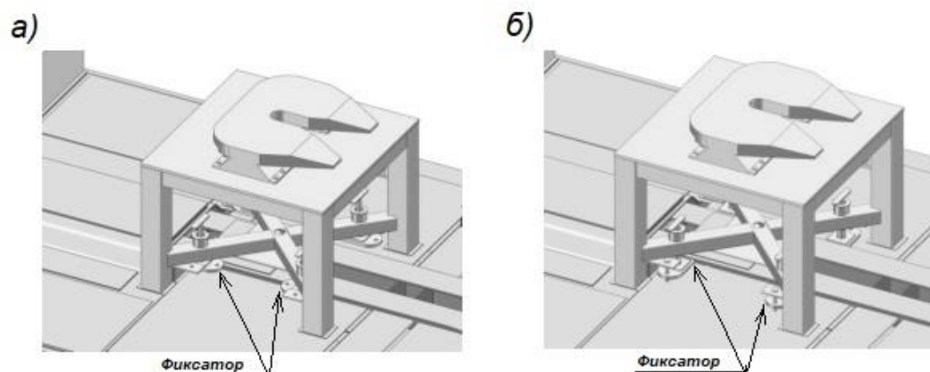
Рисунок 30 – Погрузочное и транспортное положения фиксаторов съемного сцепного устройства
