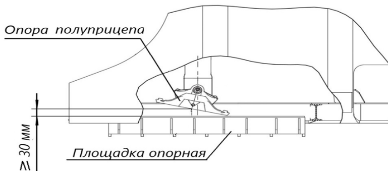
Рисунок 42 – Схема контроля положения опор полуприцепа
