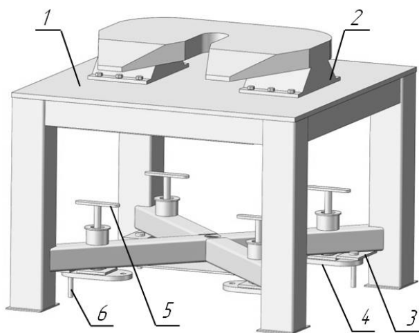
Рисунок 29 – Съемное седельное устройство
