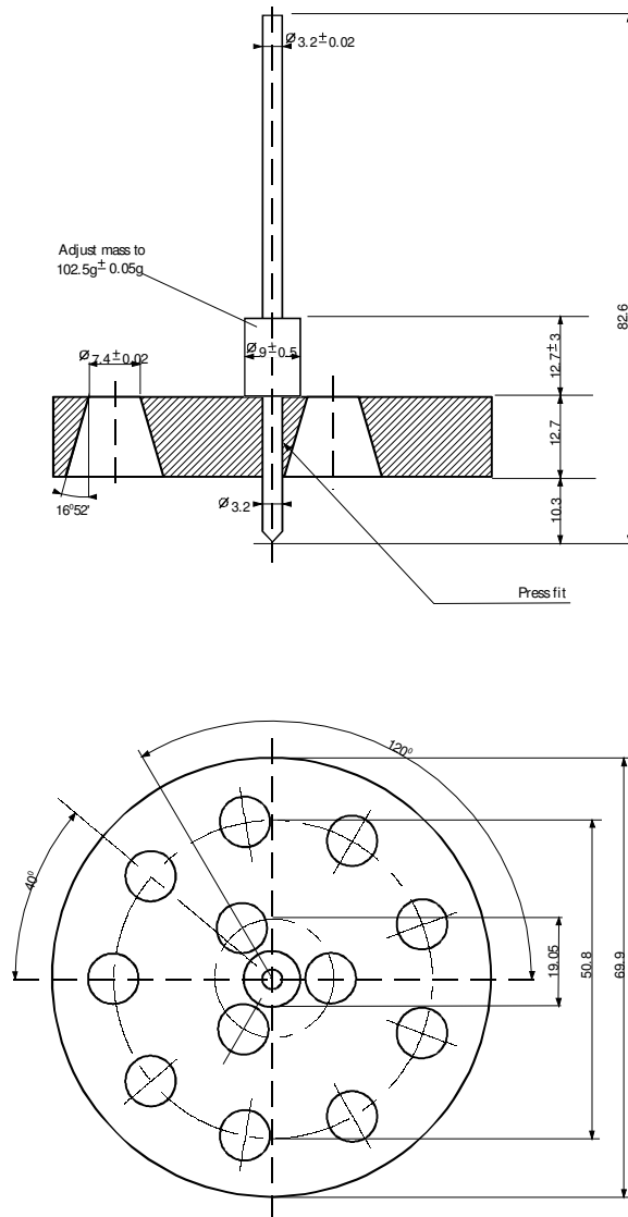
Рис. 2.4. Пенетромтр
