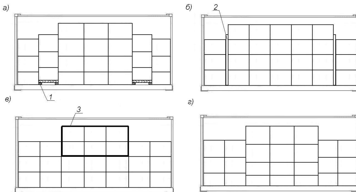
Рисунок 10 – Примеры крепления груза в неполном верхнем ярусе
