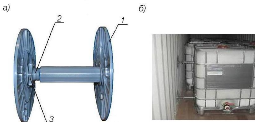
Рисунок 7 – Распорка
