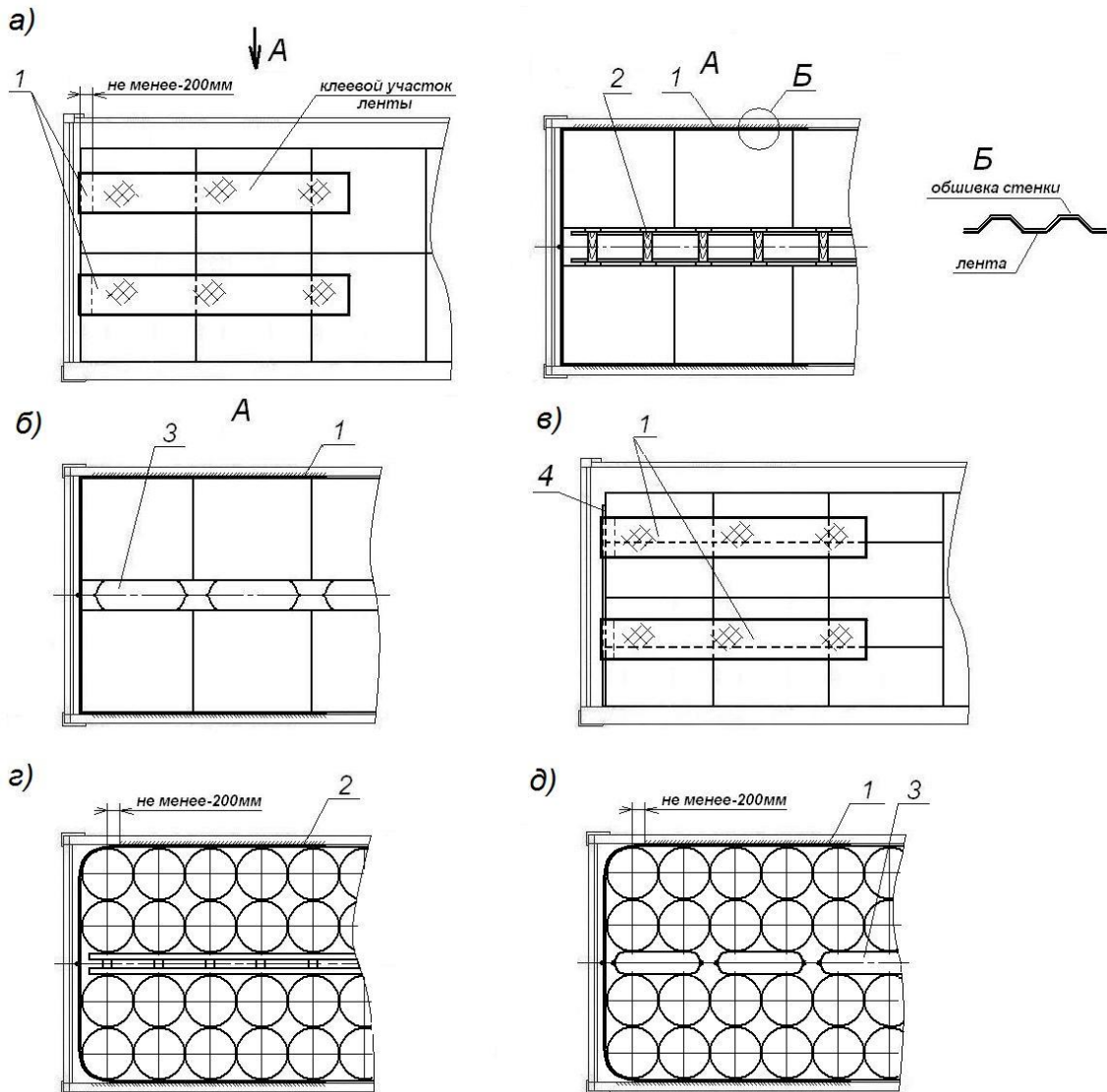
Рисунок 15 – Примеры крепления клейкой крепежной лентой а, б – крепление штабеля ящиков, коробок; г, д – крепление штабеля бочек; в – крепление с использованием экрана (щита); 1 – крепежная лента; 2 – распорная конструкция; 3 – пневмооболочка; 4 – экран (щит)
