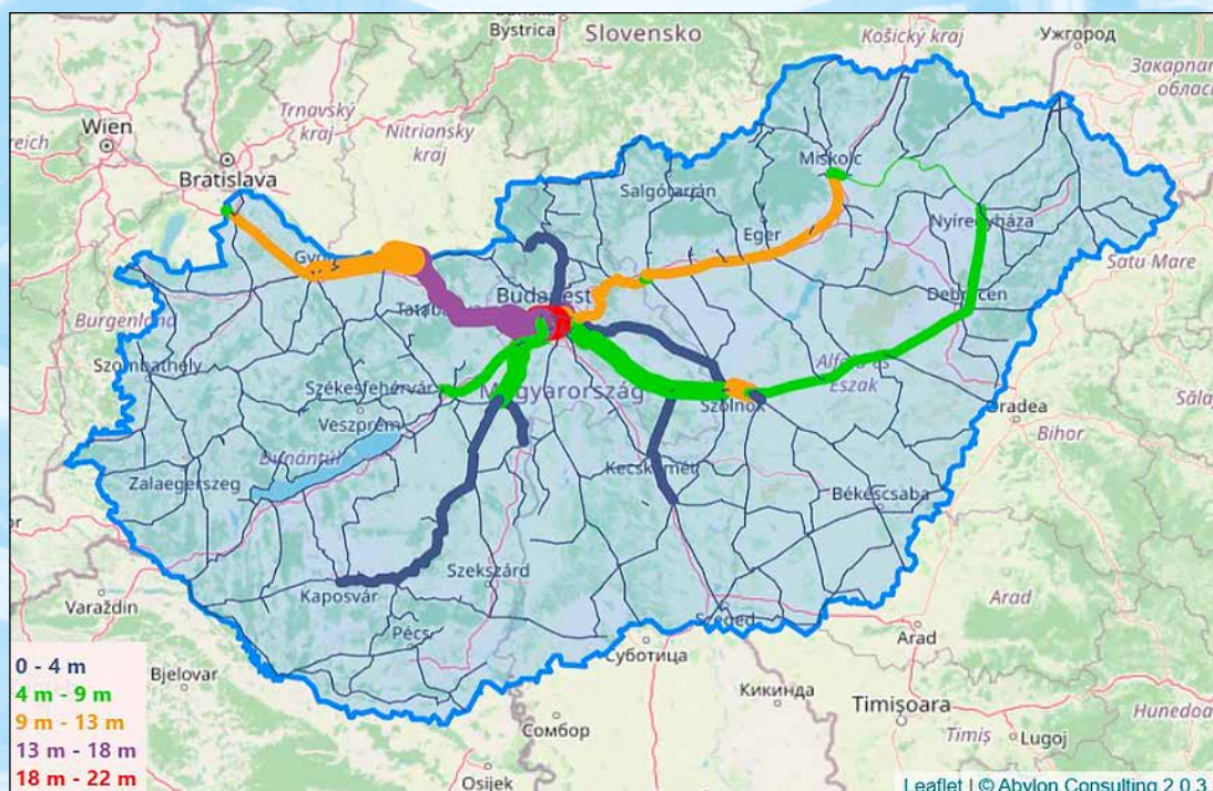
Железнодорожные линии, обеспечивающие значительную экономию выбросов углекислого газа (млн. кг)
